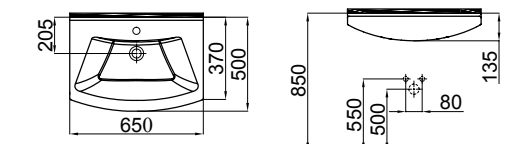
2801-0655 Vega Lavabo / Vega Washbasin (50x65)
