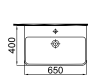
0101-0655 Dikdörtgen Lavabo / Rectangular Washbasin (40x65)
