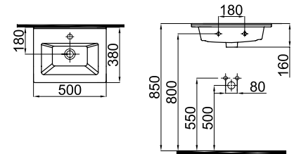
0201-4505 Merkür Lavabo / Merkur Washbasin (38x50)
