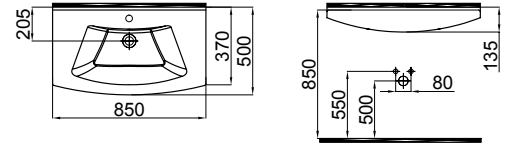
2801-0855 Vega Lavabo / Vega Washbasin (50x85)
