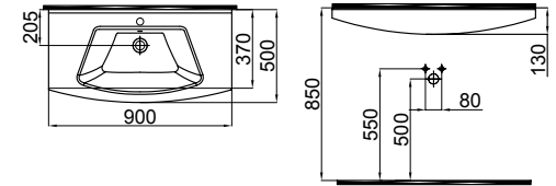
2801-0905 Vega Lavabo / Vega Washbasin (50x90)
