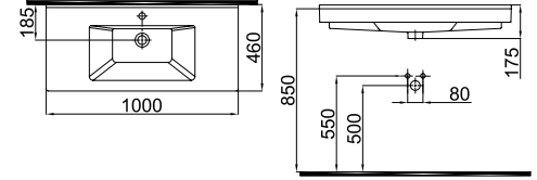
0201-5005 Merkür Lavabo / Merkur Washbasin (46x100)
